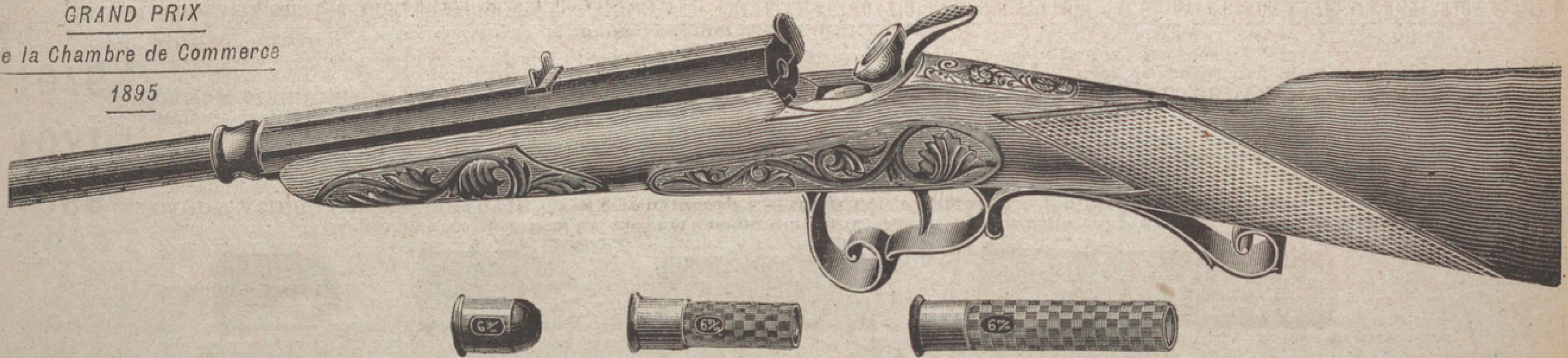
Cartouches, calibre 6 m/m, percussion annulaire, à balles et à plombs (Grandeur naturelle)
