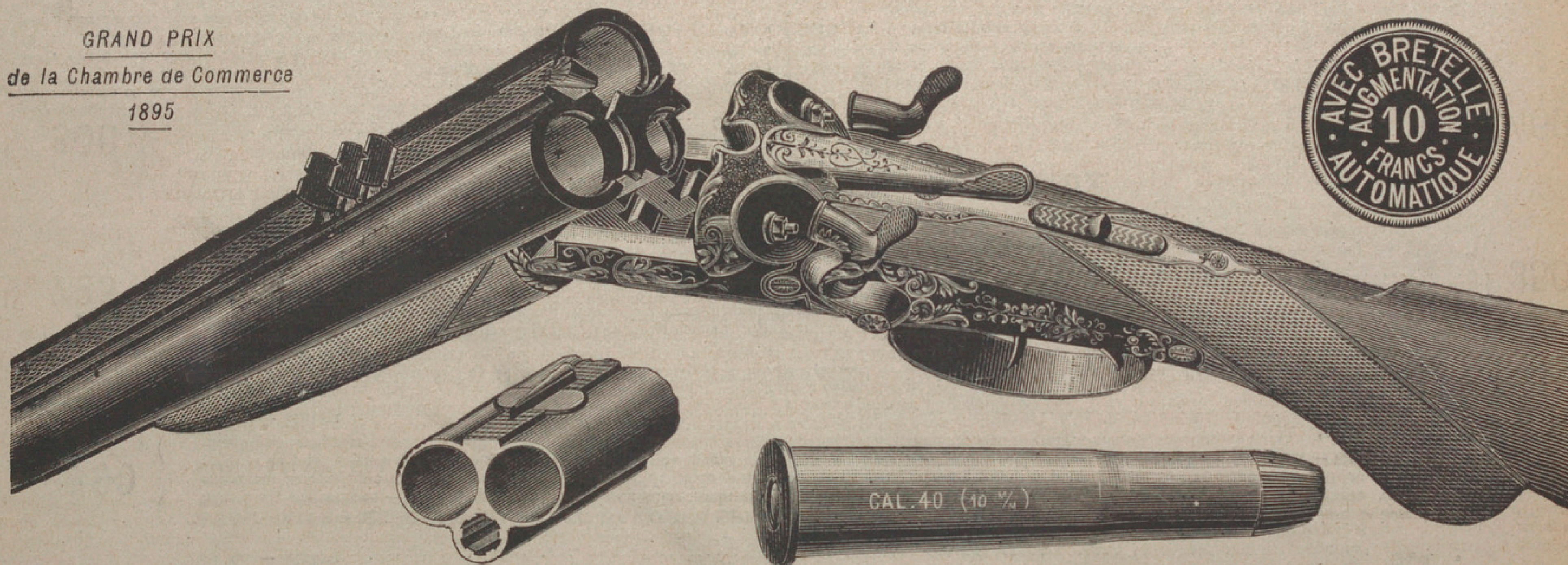
Cartouche calibre 40 (10 m/m) avec balle pleine ou Express
