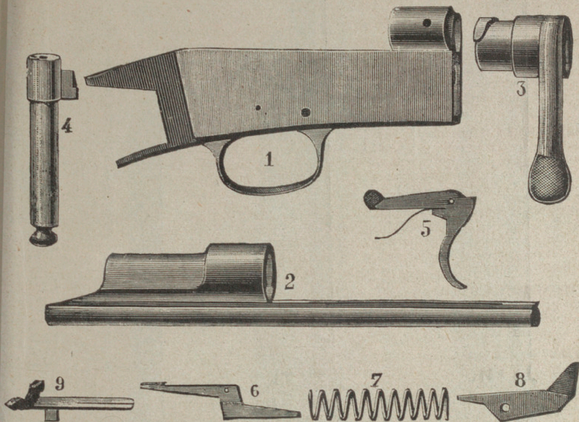
1 Boîte de culasse. — 2 Culasse mobile — 3 Tête mobile — 4 Marteau percuteur — 5 Détente — 6 Gâchette — 7 Ressort — 8 Pièce d'arrêt — 9 Extracteur.
