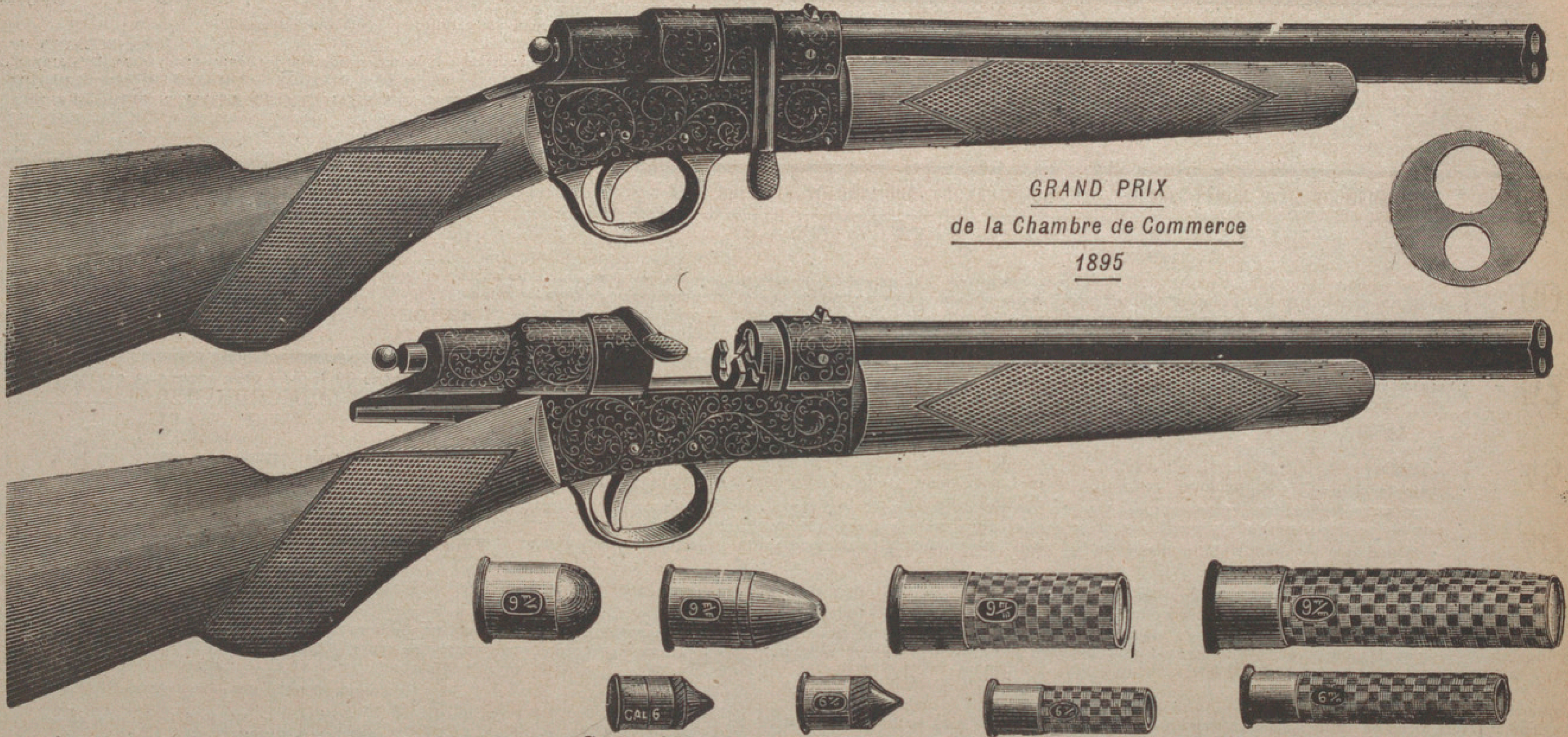
Cartouches calibres 6 et 9 m /m, percussion annulaire, à balle et à plombs ( Grandeur naturelle )
